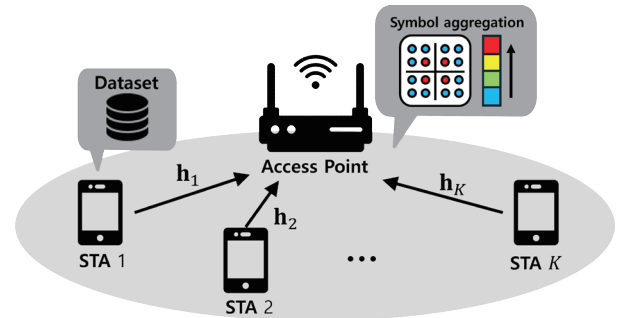
그림 1. STLC 기반 디지털 AirComp 시스템 모델
